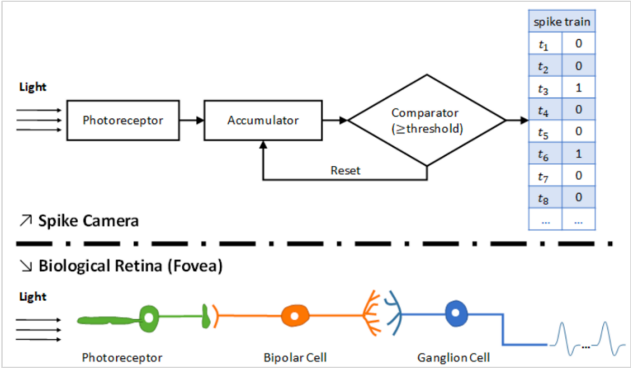
图 3.3 脉冲摄像头[4]
