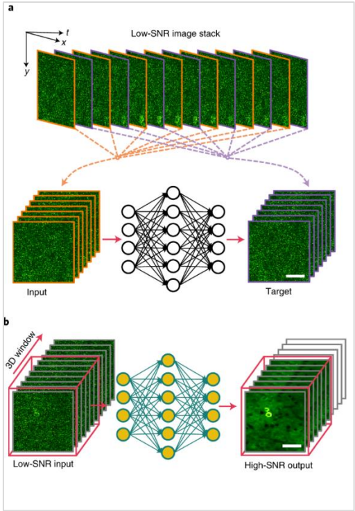
图 5.10 a) DeepCAD 自监督训练示意图。模型训练过程中不需要高信噪比信号。只需要将原始的低信噪比延时成像中取出固定时间窗口长度的图栈。将该图栈相互间隔的划分的两个子栈。分别当作输入数据和目标数据来训练一个 3D U-Net 神经网络。训练后的该网络即具有滤噪功能。b) 训练好的 DeepCAD 实际运行效果[16]。
