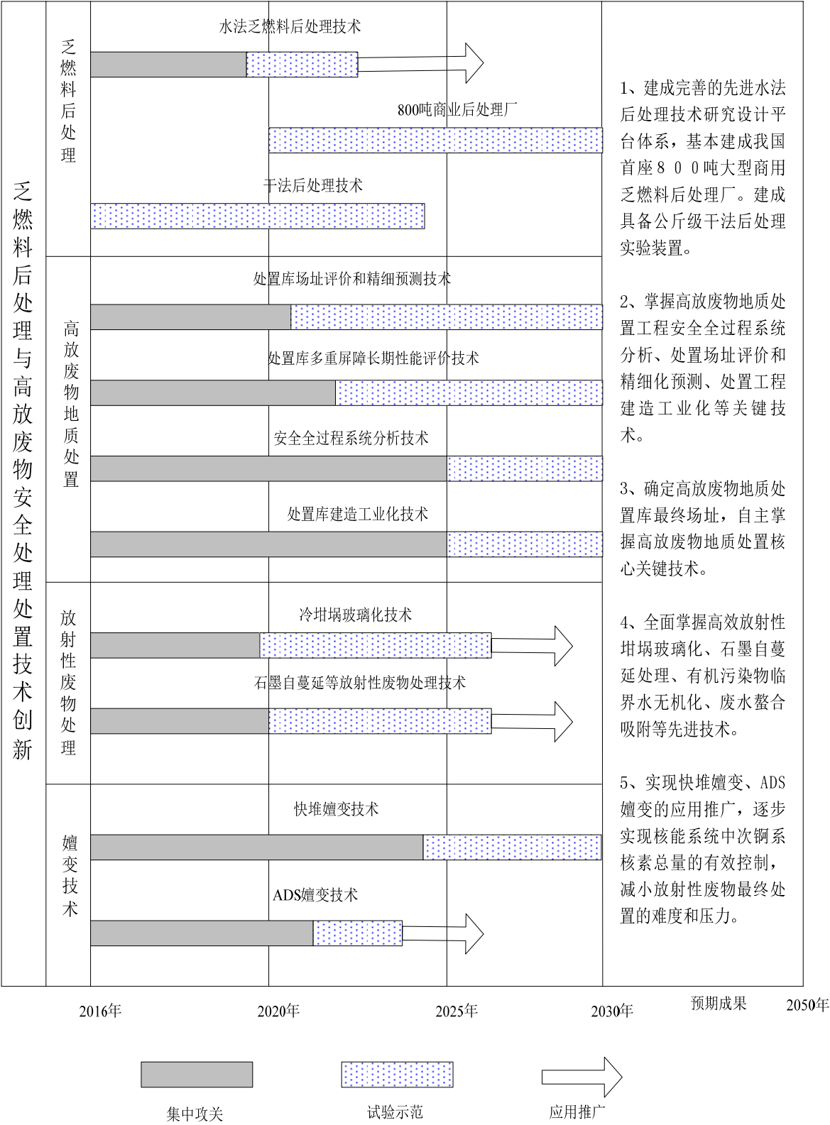
乏燃料后处理与高放废物安全处理处置技术创新路线图
