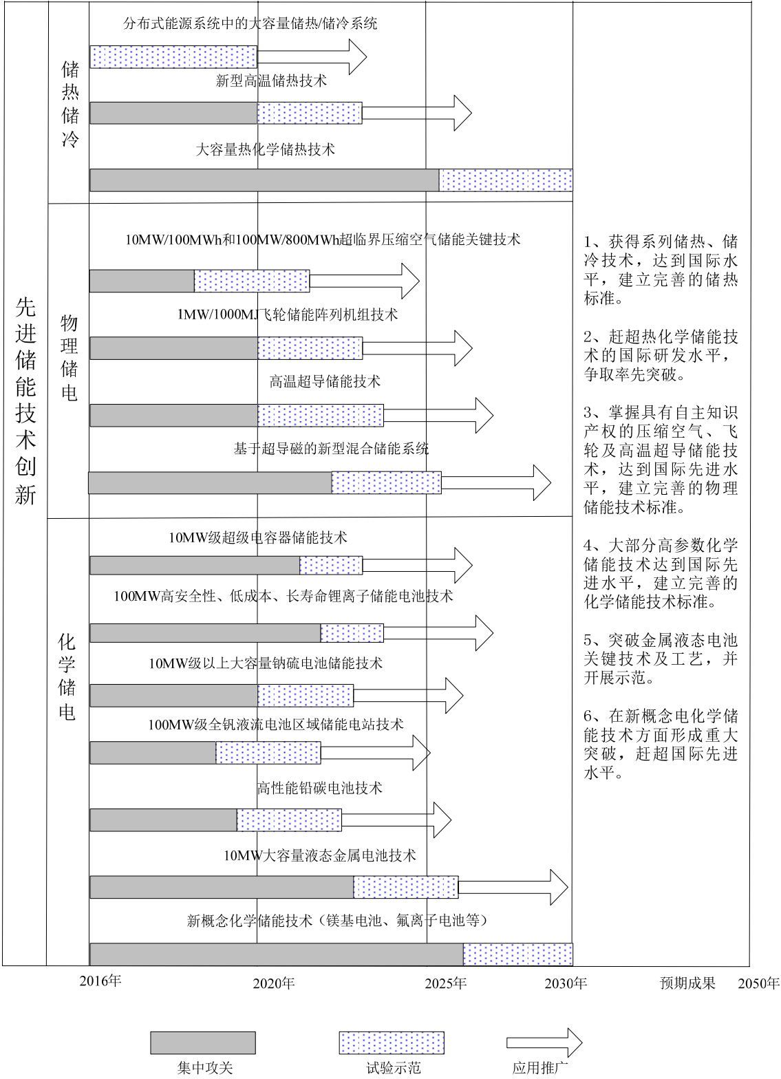
先进储能技术创新路线图
